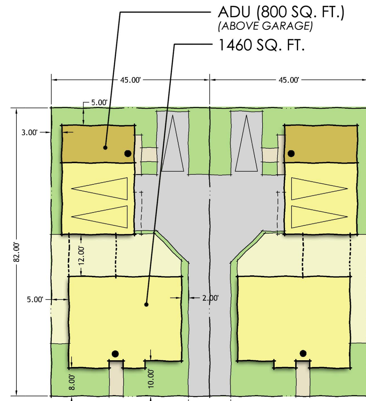
COTTAGE DUETS (CD1)
