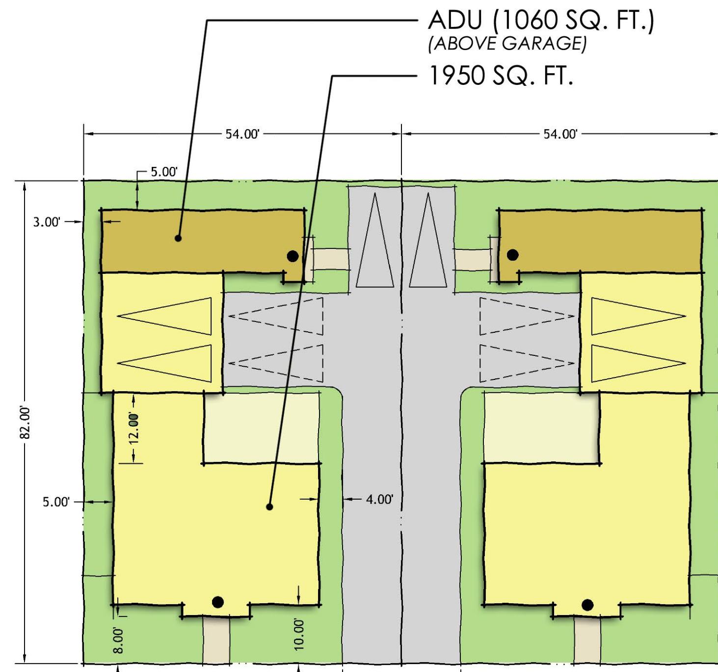
COTTAGE DUETS (CD2)
